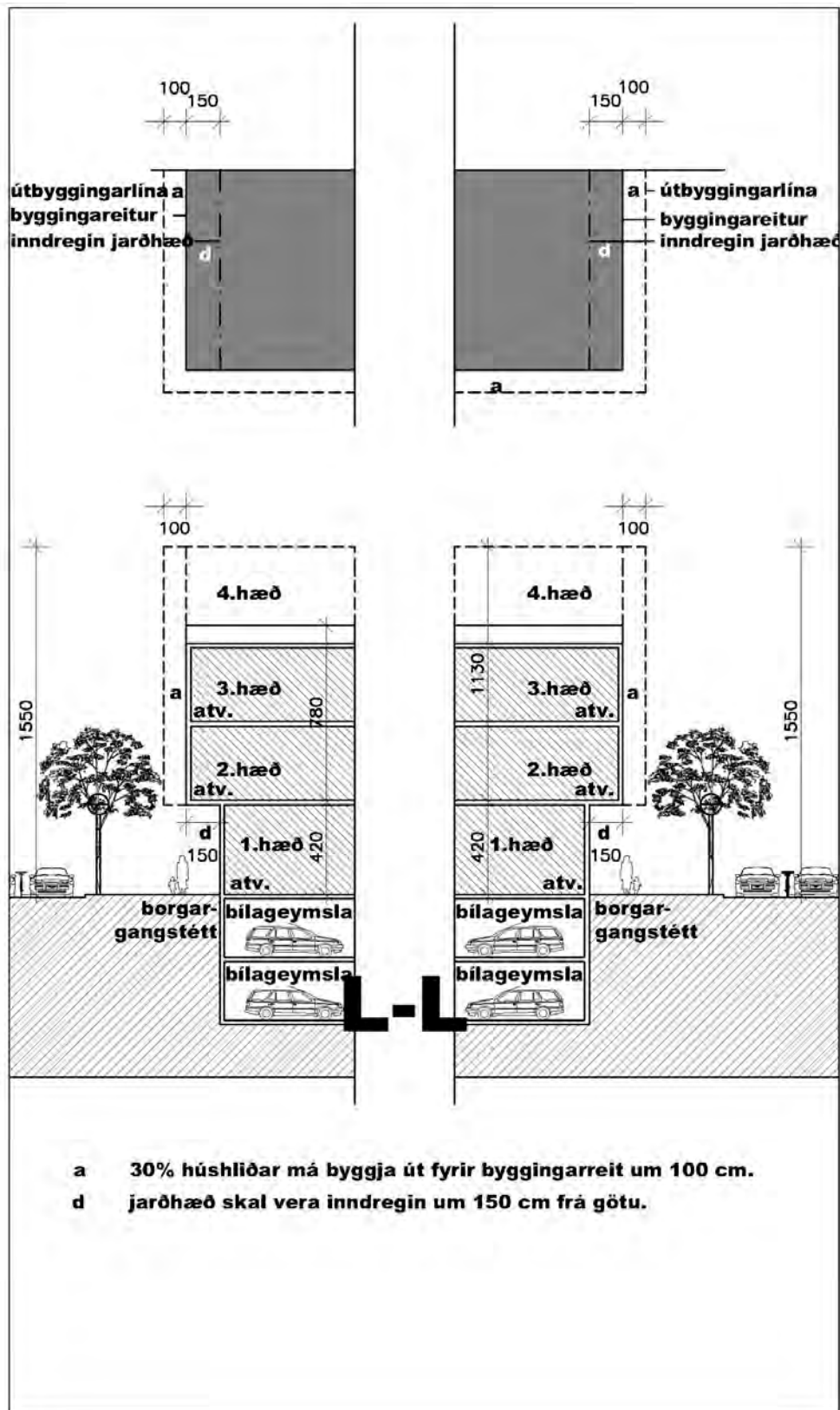
Skilmálasnið L-L
