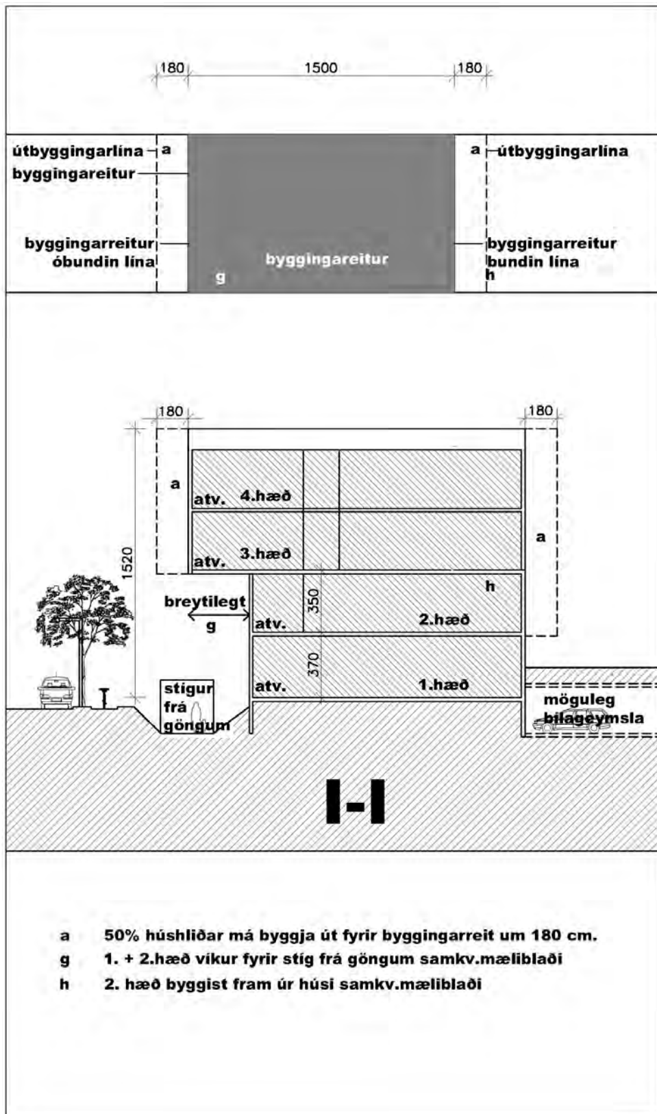
Skilmálasnið I-I
