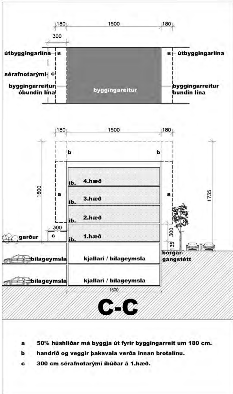
Skilmálasnið C-C
