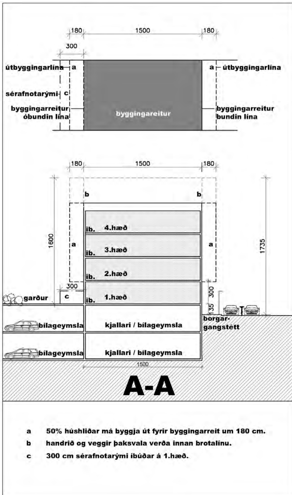
Skilmálasnið A-A
