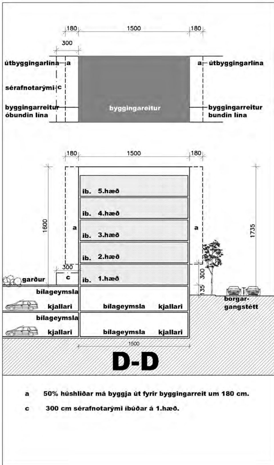
Skilmálasnið D-D
