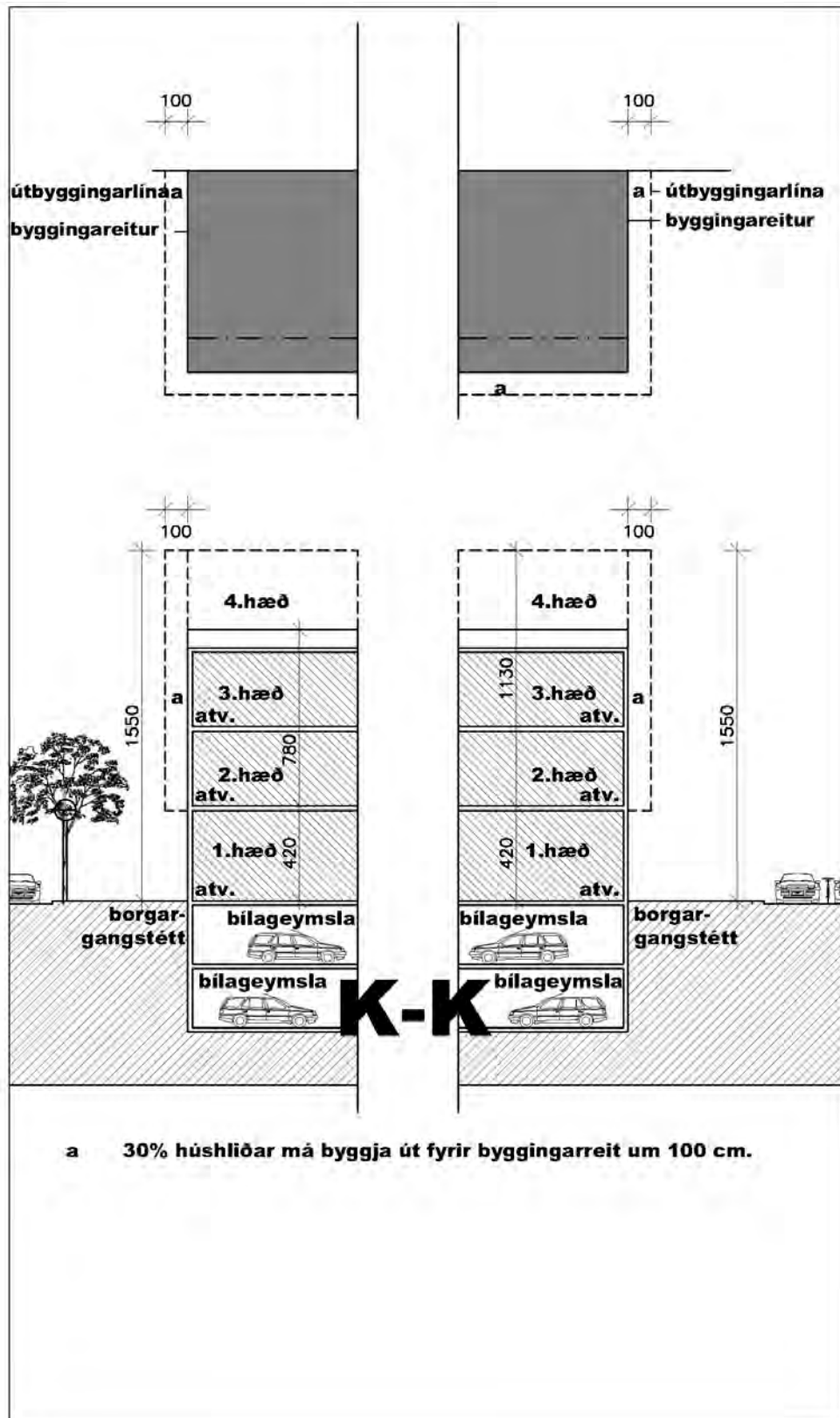
Skilmálasnið K-K
