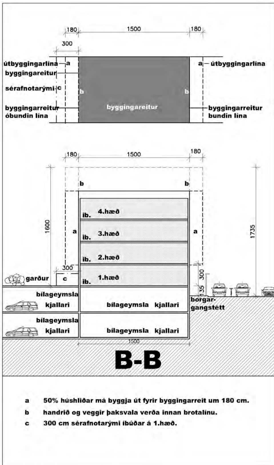
Skilmálasnið B-B
