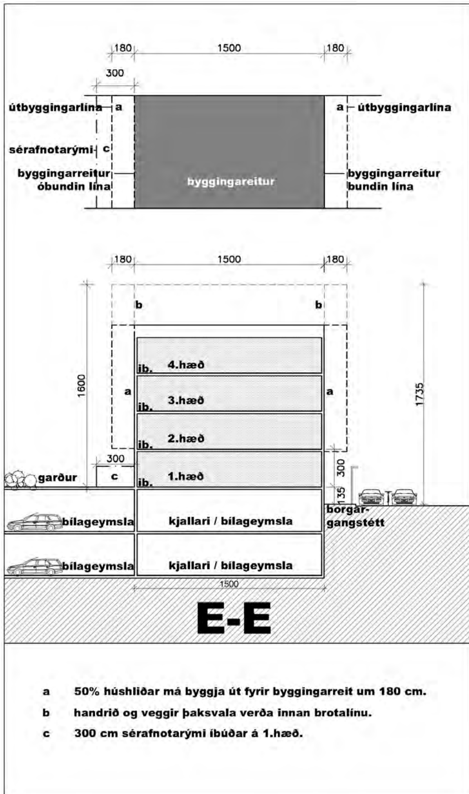
Skilmálasnið E-E
